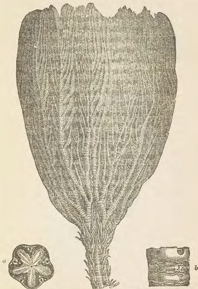
PENTACRINUS FASCICULOSUS. (Lias.)
